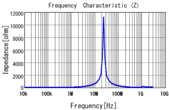
■ 1255AY-100M |Z|
