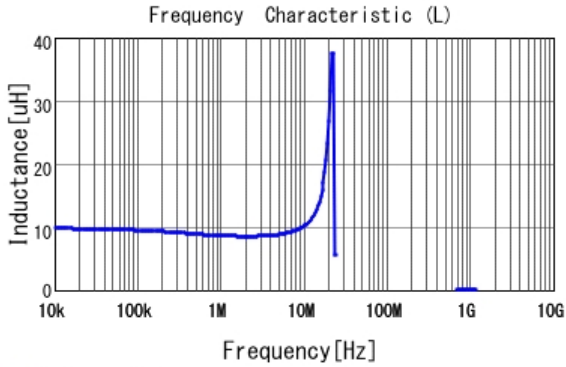
■ 1255AY-100M L
