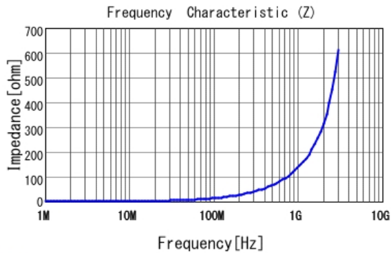
■ LQW15AN22NG8Z |Z|
