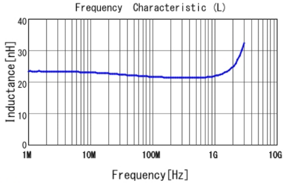
■ LQW15AN22NG8Z L
