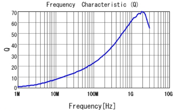
■ LQW15AN22NG8Z Q
